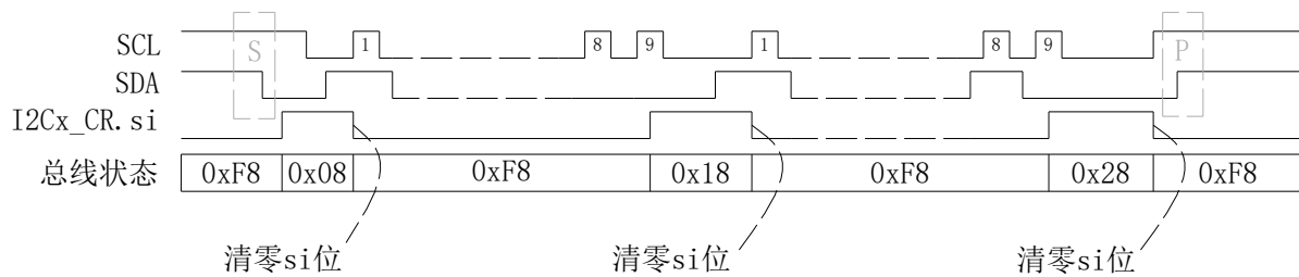
图 7-7 主发送模式数据同步图
