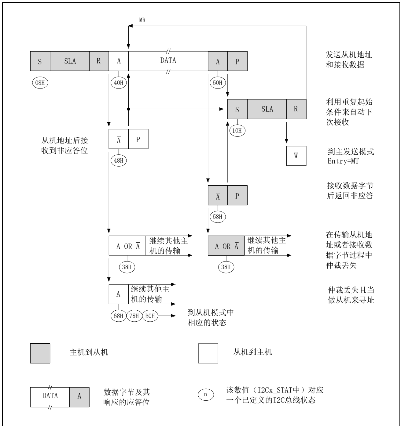
图 7-10 I2C 主机接收状态图
