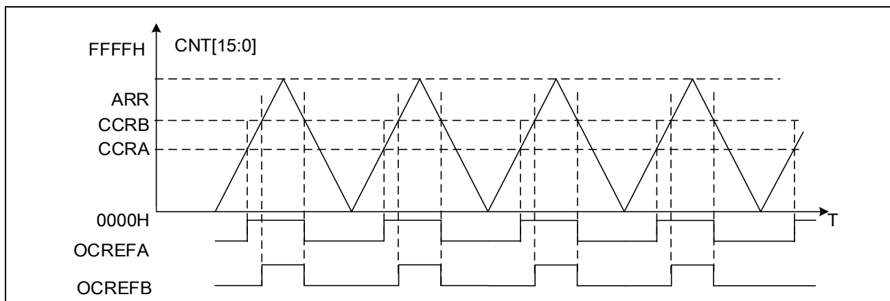
图 14-35 三角波计数双点比较 OCREF 输出 (OCM x =111)
