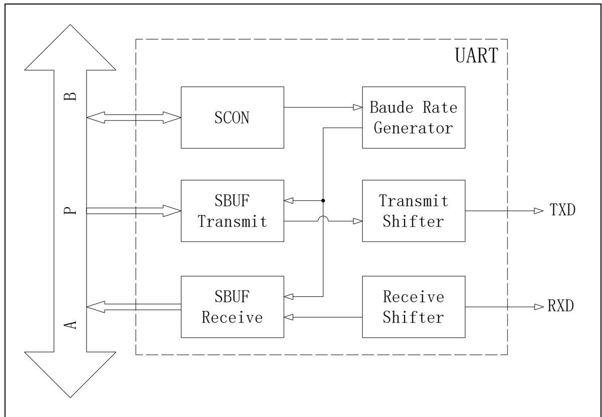
图 18-1 结构框图
