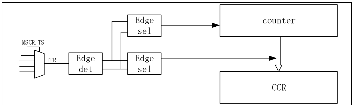
图 14-9 PWC测量框图
