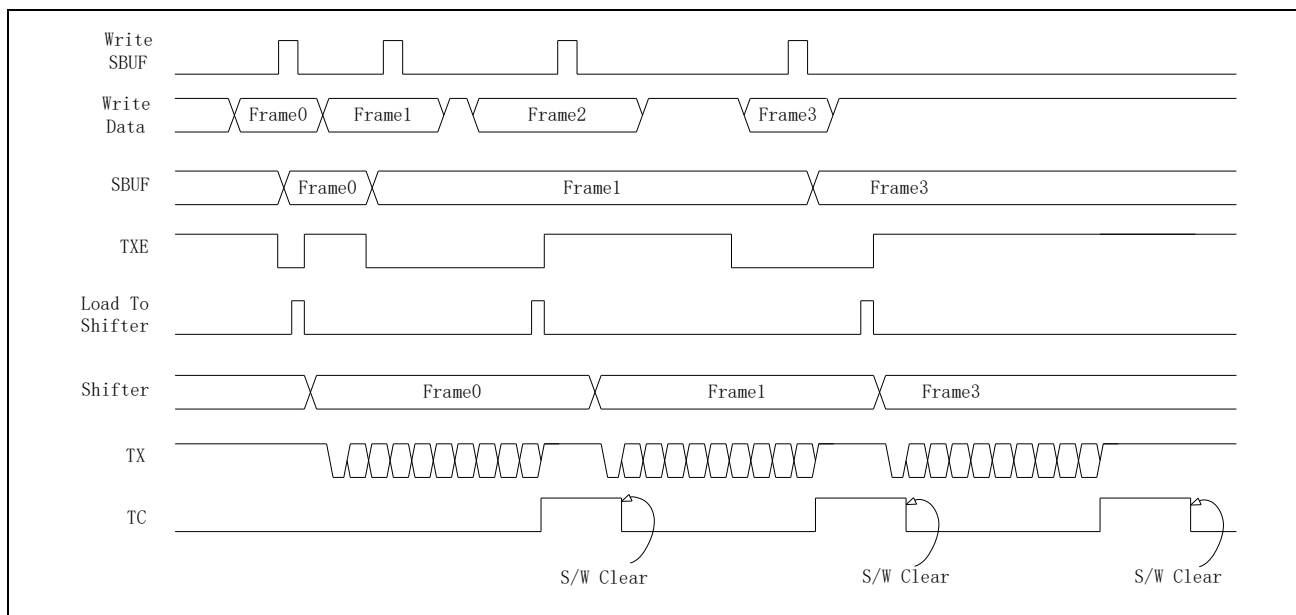
图 18-14 发送缓存
