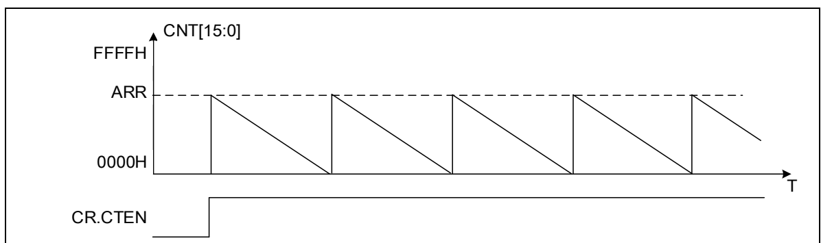
图 14-20 边沿对齐计时器波形(DIR =1)
